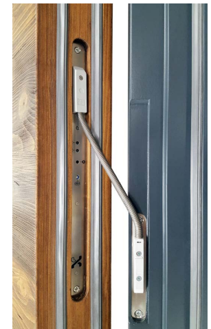
Steckbarer Kabelübergang
